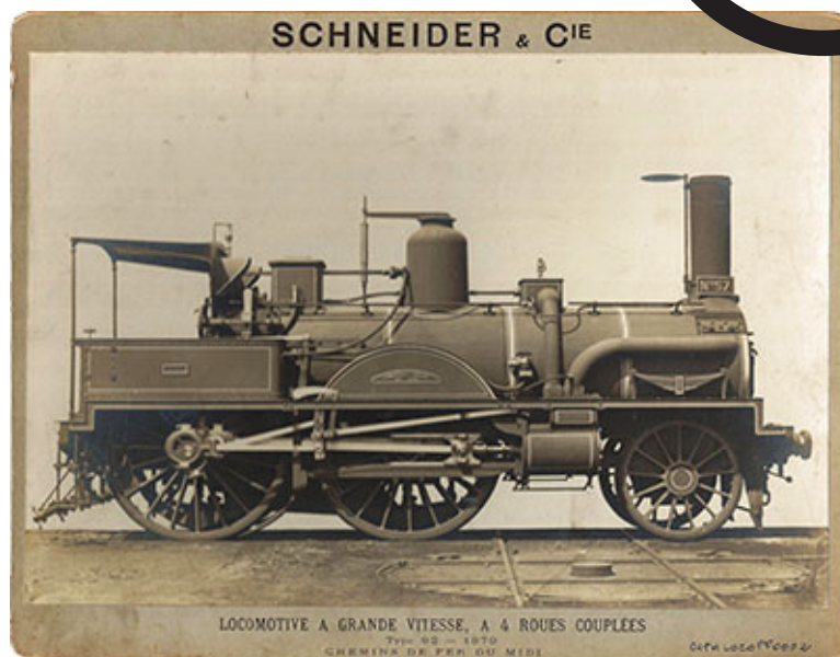
Locomotive à vapeur compound à 4 roues couplées fabriquée par Schneider et Compagnie aux usines du Creusot en 1879 pour le Chemin de fer du Midi
