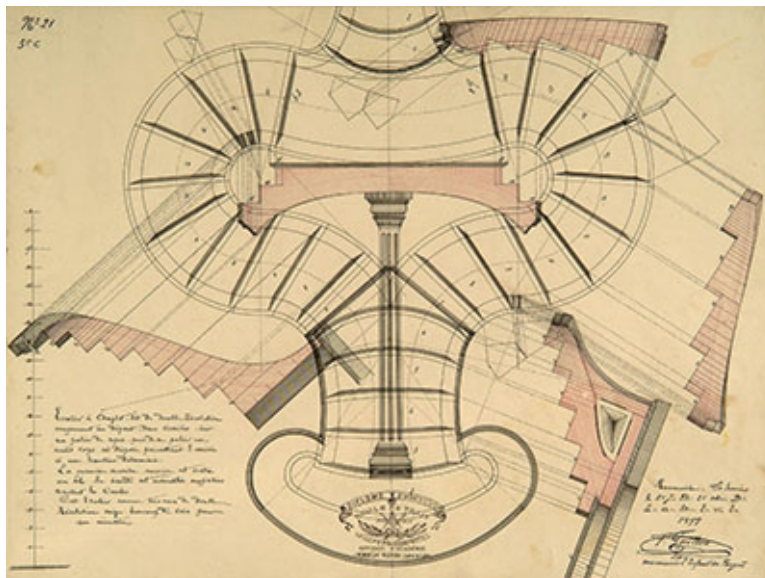
Épure de tracé de charpente (fin du XIX e siècle)
